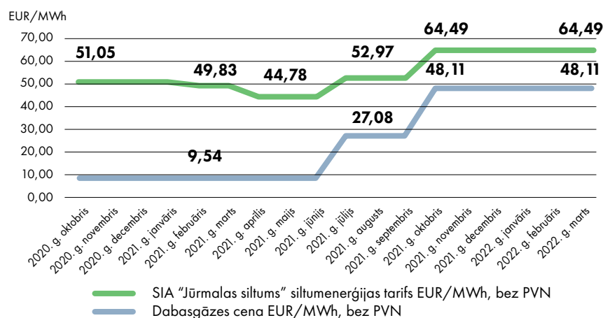
SIA "Jūrmalas siltums" tarifs attiecībā pret dabasgāzes cenu EUR/MWh
