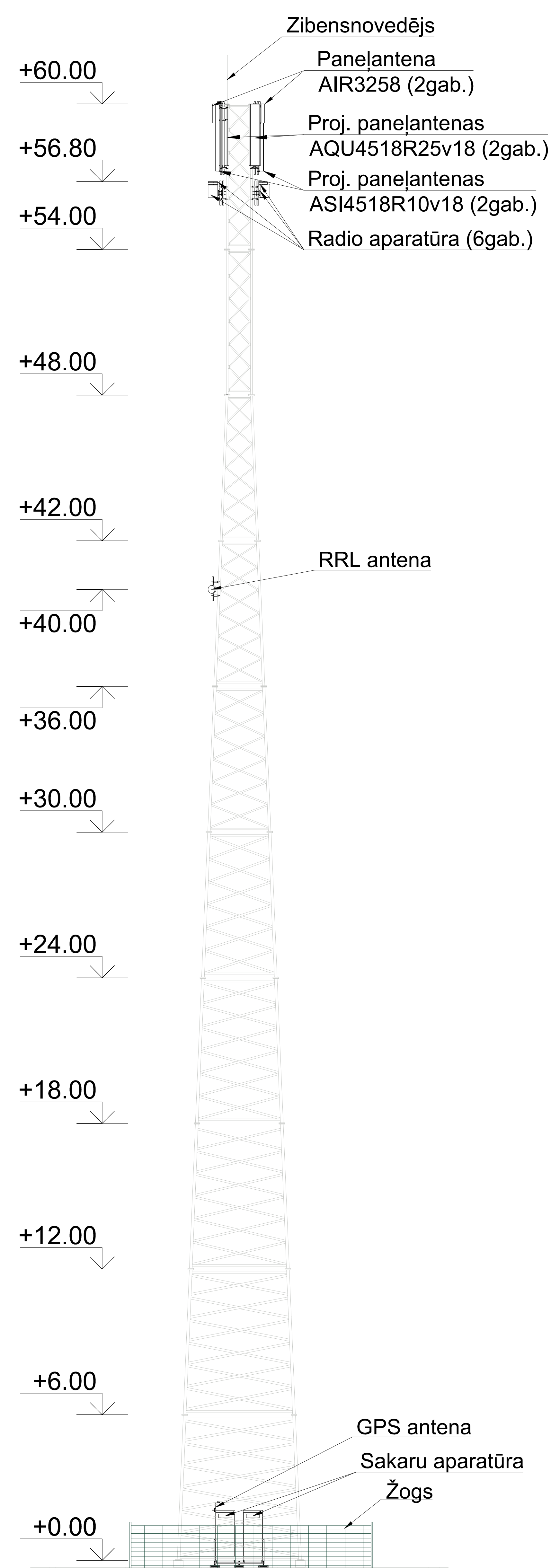
FASĀDE M1:100
