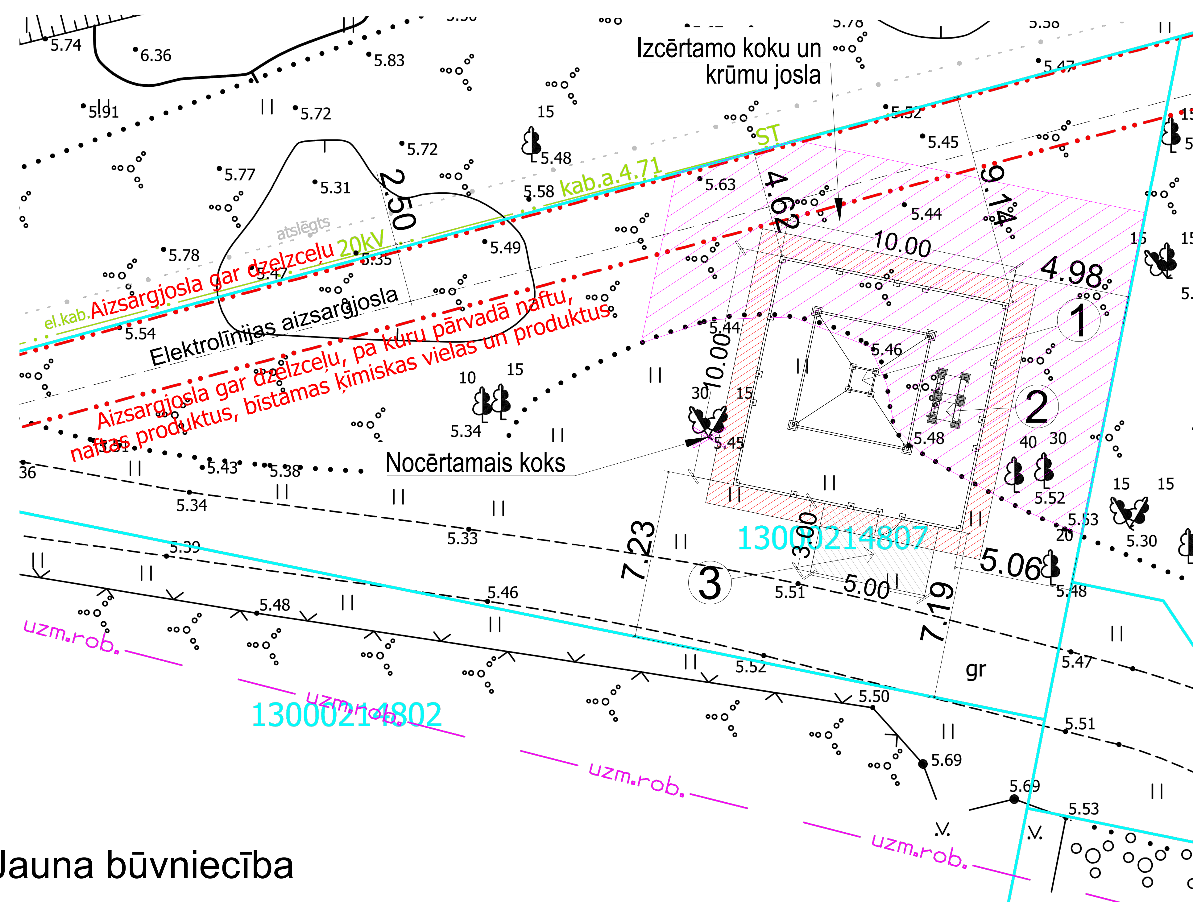
PLĀNS M1:100
